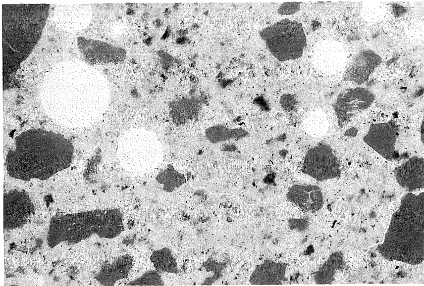
Figur 16. Snit i beton med relativ lav kapillarporøsitet, svarende til et v/c -forhold på ca. 0,55-0,60. Billedet er taget i et fluorescensmikroskop. Udsnittet er ca. 1,5 \times 1,0 mm. Foto: COWIconsult.
