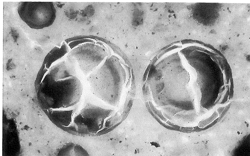
Figur 13. Snit af beton, støbt med kompakteret mikrosilica. Manglende dispergering har medført mikrosilicaklumper i kitmassen. Mikrosilica er alkalireaktiv og kan reagere med kitmassens porevæske. Der er dannet revner, både i og ud fra klumperne. Billedet er taget i et fluorescensmikroskop. Udsnittet er ca. 0,5 \times 0,4 mm. Foto: AEC.
