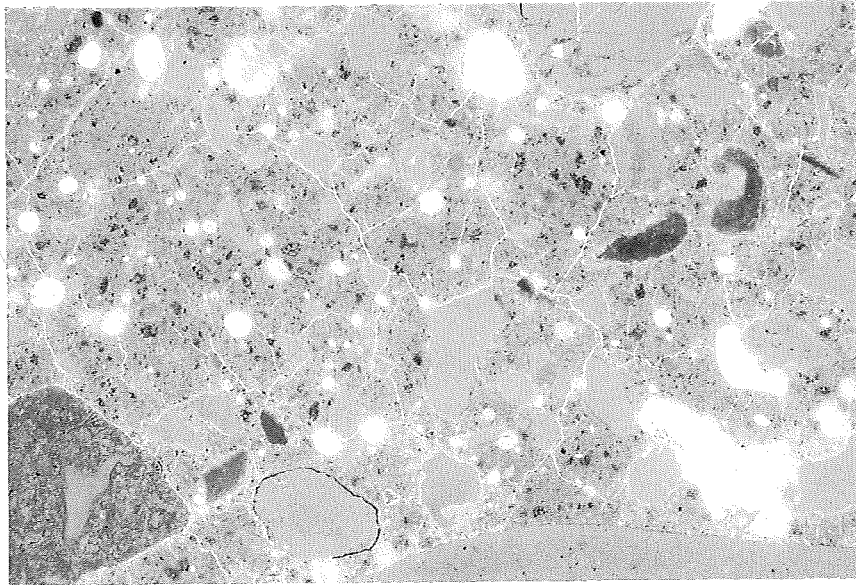
Figur 21. Snit i beton med stor intensitet af mikrorevner (revnevidde under 0,01 mm) i form af såvel pasta- som vedhæftningsrevner. Billedet er taget i fluorescensmikroskop. Udsnittet er ca. 1,5 × 1,0 mm. Foto: COWIconsult.
