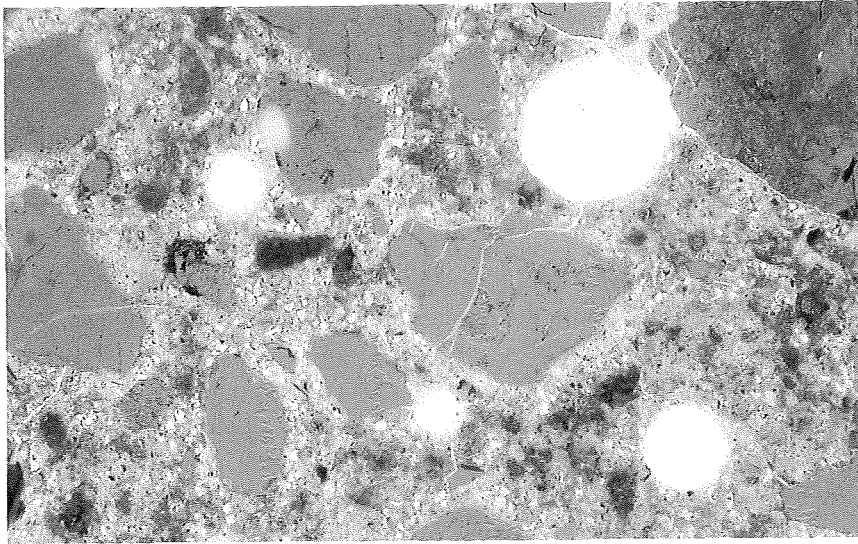
Figur 15. Snit i beton med relativ lav kapillarporøsitet, svarende til et v/c -forhold på ca. 0,40. Billedet er taget i et fluorescensmikroskop. Udsnittet er ca. 1,5 \times 1,0 mm. Foto: COWIconsult.
