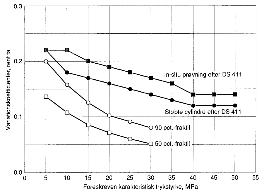
Figur 12. Variationskoefficienter, målt af Dansk Fabriksbetonkontrol i 1982. Der er anvendt følgende signaturer: ○ er 90 pct.-fraktile. □ er 50 pct.-fraktile. ● er den udokumenterede variationskoefficient for støbte prøvecylindre efter DS 411. ■ er den udokumenterede variationskoefficient for in-situ prøvning efter DS 411. Kilde: Dansk Fabriksbetonkontrol 1982.
