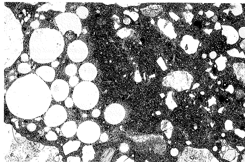
Figur 17. Snit i luftindblandet beton, hvor luftboblerne har tydelig tendens til at klumpe sig sammen. Billedet er taget i polarisationsmikroskop med parallelle nicoller. Udsnittet er ca. 1,5 × 1,0 mm. Foto: COWIconsult.
