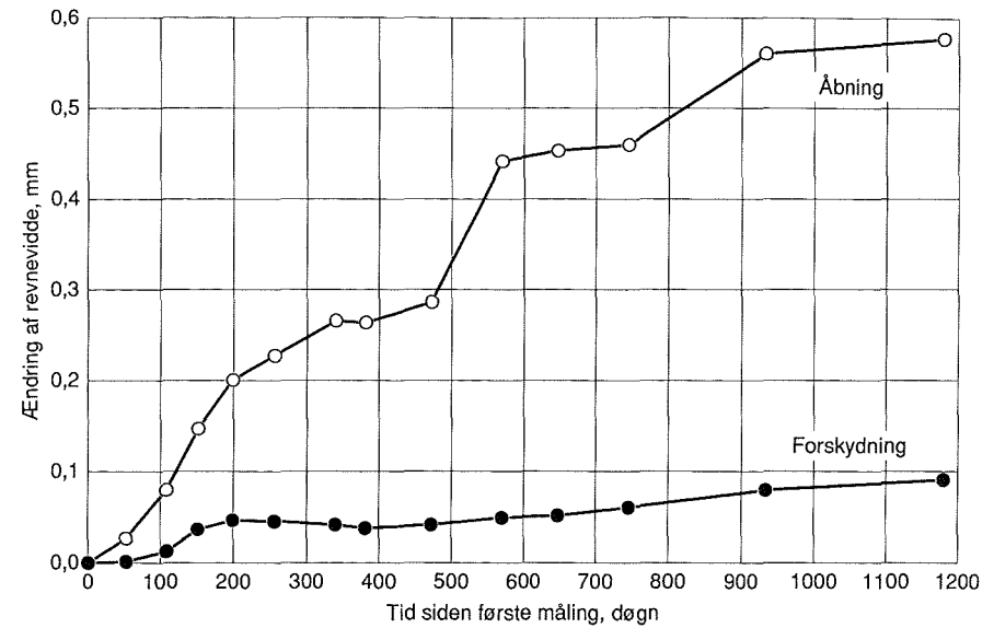
Figur 4. Eksempel på graf for en revnes viddeændring og forskydning versus tid, målt med en 3-punkts målerose, jf. figur 2. Her er der registreret stor åbning og lille forskydning, sml. figur 5. Revnen skyldes igangværende alkalireaktion. Bemærk sæsonsvingningerne. Kilde: AEC.
