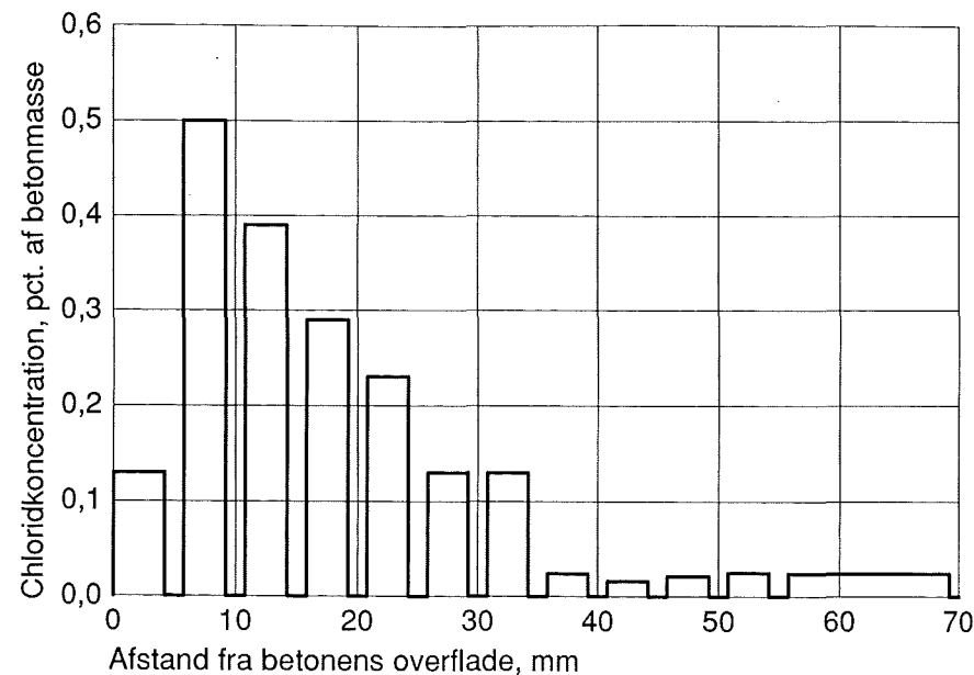
Figur 24. Chloridprofil i et område af et rammeelement beton, hvor der er korroderet armering. Chloridprofilen har det typiske forløb, som kendes fra beton, hvor chlorid er trængt ind fra overfladen og hvor overfladen er carbonatiseret og eventuelt udvasket. Det ses, at chloridindholdet i betonen nær armeringen er større end det, der betragtes som kritisk, dvs. korrosionsfremkaldende ved tilstedeværelse af fugt og ilt. Kilde: AEC.
