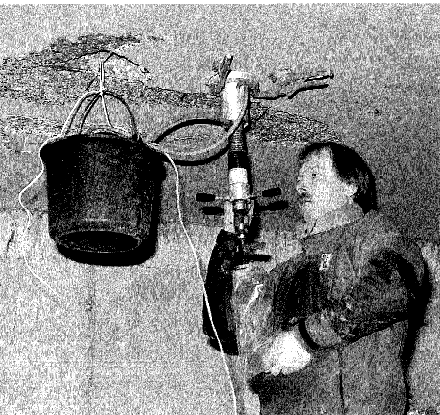
Figur 8. For de fleste betonundersøgelser i Danmark vil det være tilstrækkeligt at basere betonundersøgelsen på Ø75 mm borekerner. Derved kan man anvende et boreudstyr, som er let at montere, håndtere og transportere. Foto: AEC.
