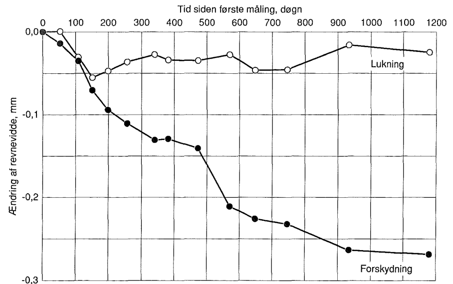
Figur 5. Eksempel på graf for en revnes viddeændring og forskydning versus tid, målt med en 3-punkts målerose, jf. figur 2. Her er der registreret lille lukning og stor forskydning, sml. figur 4. Revnen skyldes igangværende alkalireaktion. Bemærk sæsonsvingningerne. Kilde: AEC.
