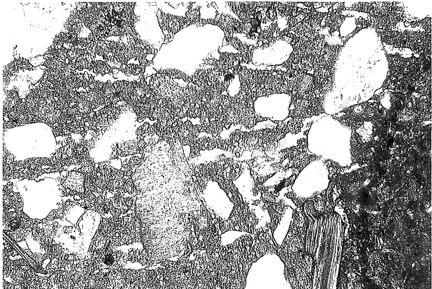
Figur 19. Typisk revnebillede i snit af beton, der har været udsat for frost før hærkning. Billedet er taget i polarisationsmikroskop med parallelle nicoller. Udsnittet er ca. 1,5 \times 1,0 mm. Foto: COWIconsult.
