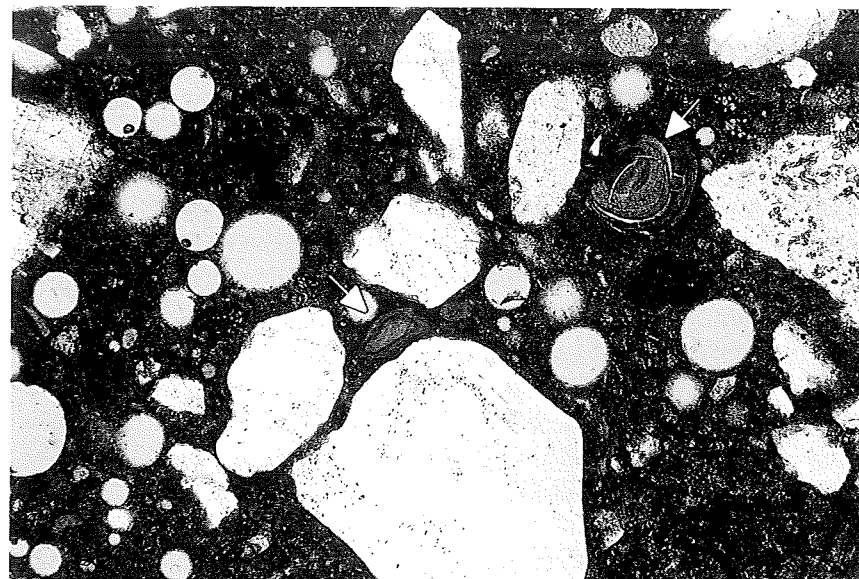
Figur 14. Snit i beton med klumper af udispergeret mikrosilica (ved pile). Billedet er taget i polarisationsmikroskop med parallelle nicoller. Udsnittet er ca. 1,5 \times 1,0 mm. Foto: COWIconsult.
