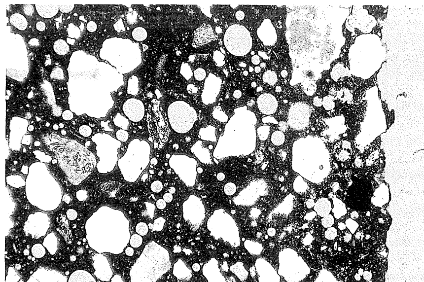
Figur 18. Snit i luftindblandet beton med middellindhold af kugleformede luftbobler. Luftboblerne er ensformigt fordelt i betonens kitmasse. Billedet er taget i et polarisationsmikroskop med parallelle nicoller. Udsnittet er ca. 5 × 3 mm. Foto: COWIconsult.
